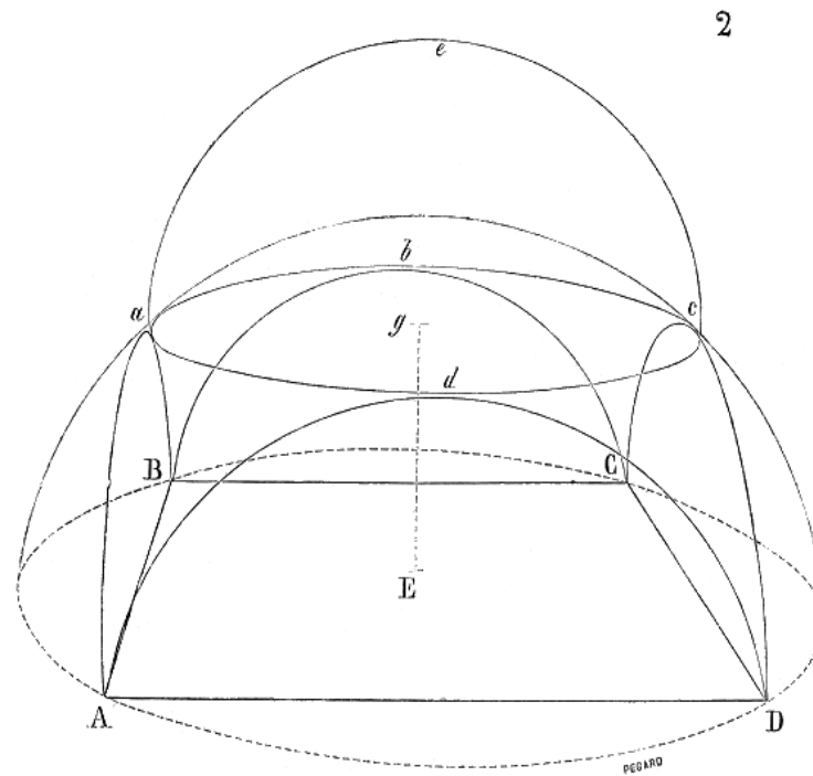
Coupole sur pendentif
